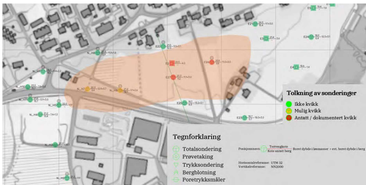
Figur 6: Antatt avgrensning av sensitive masser (utklipp V101 fra 19028-RIG01)
