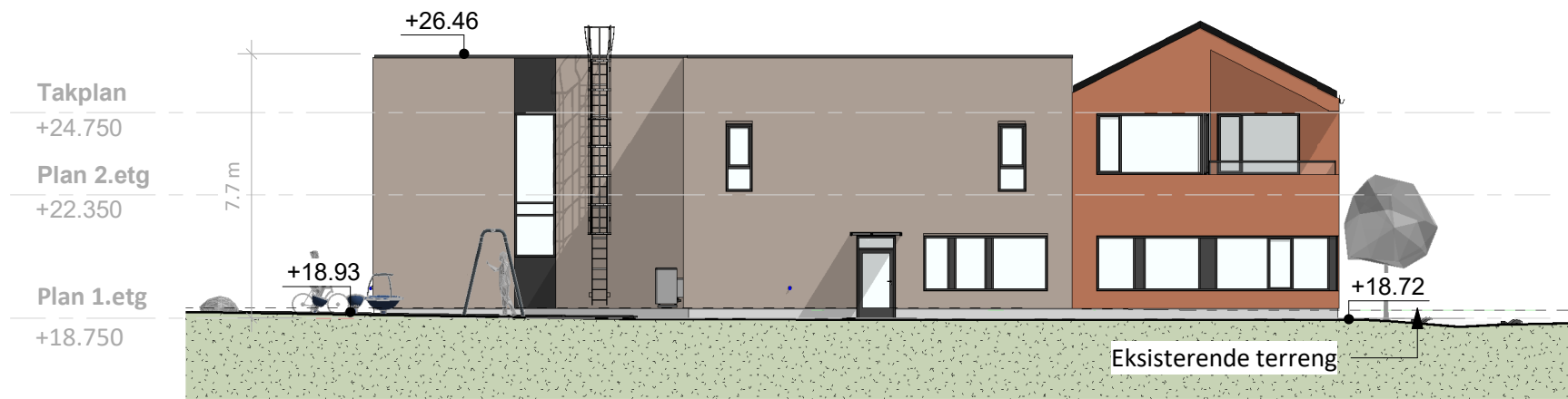
Fasade Vest
