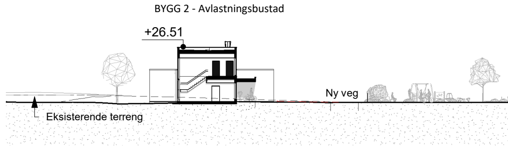
Snitt T3 R
