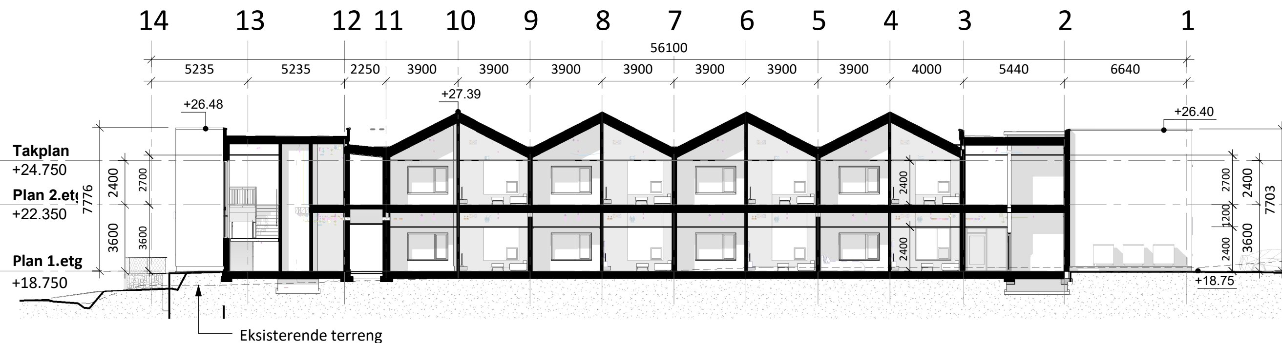
Snitt B
