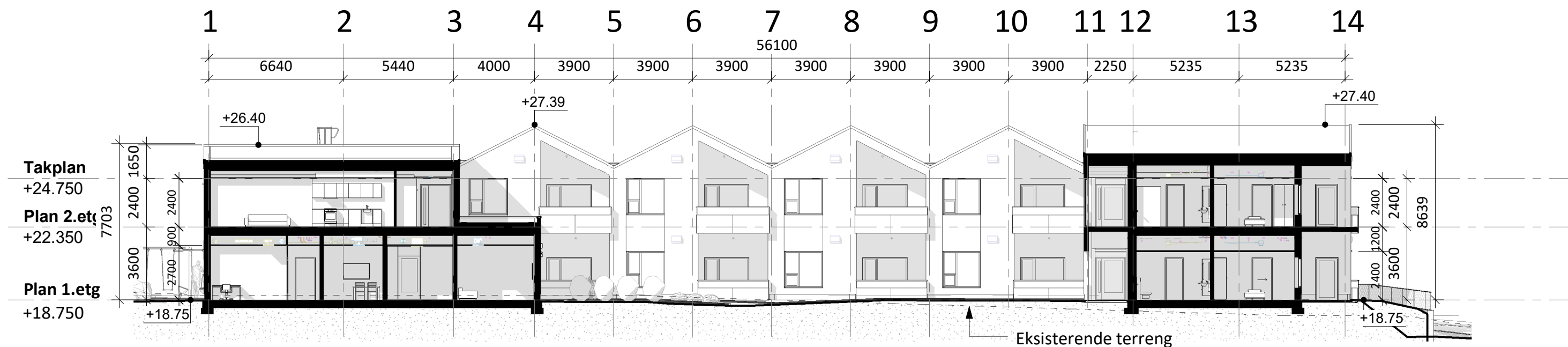
Snitt A
